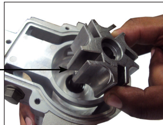
Rotor
